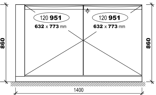
Doppeltüre 1400 - (BREITER)
